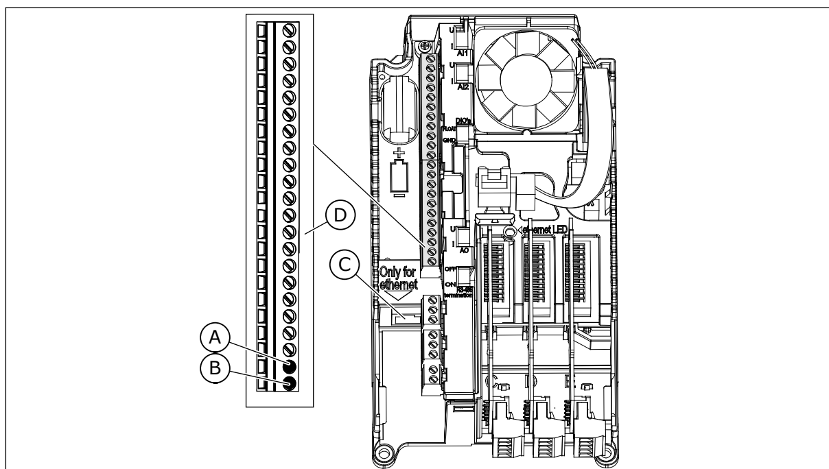
Рис. 41: Разъемы Ethernet и RS485
