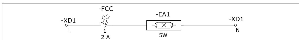
Рис. 17: Освещение шкафа
