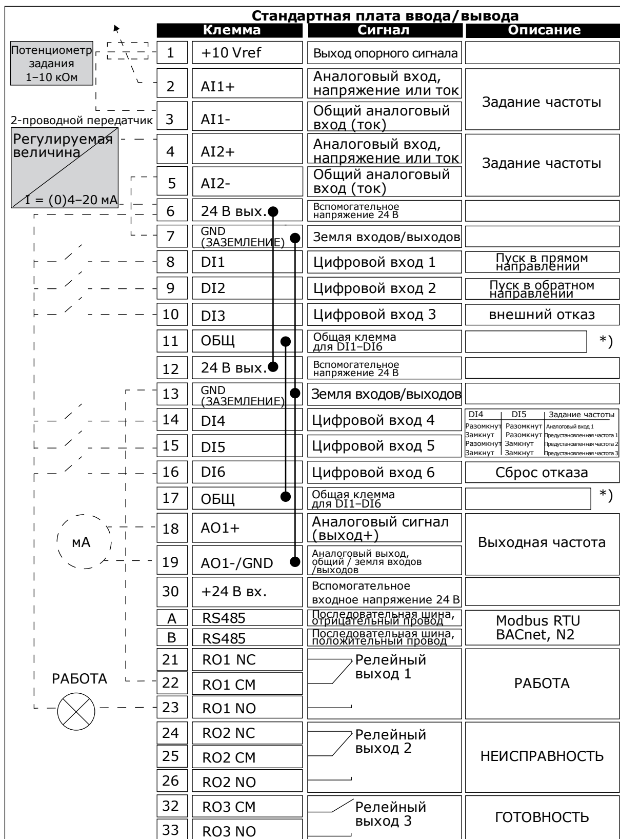
Рис. 37: Сигналы клемм управления привода на стандартной плате ввода/вывода и пример подключения. При заказе с дополнительным кодом +SBF4 релейный выход 3 замещается входом термистора.
