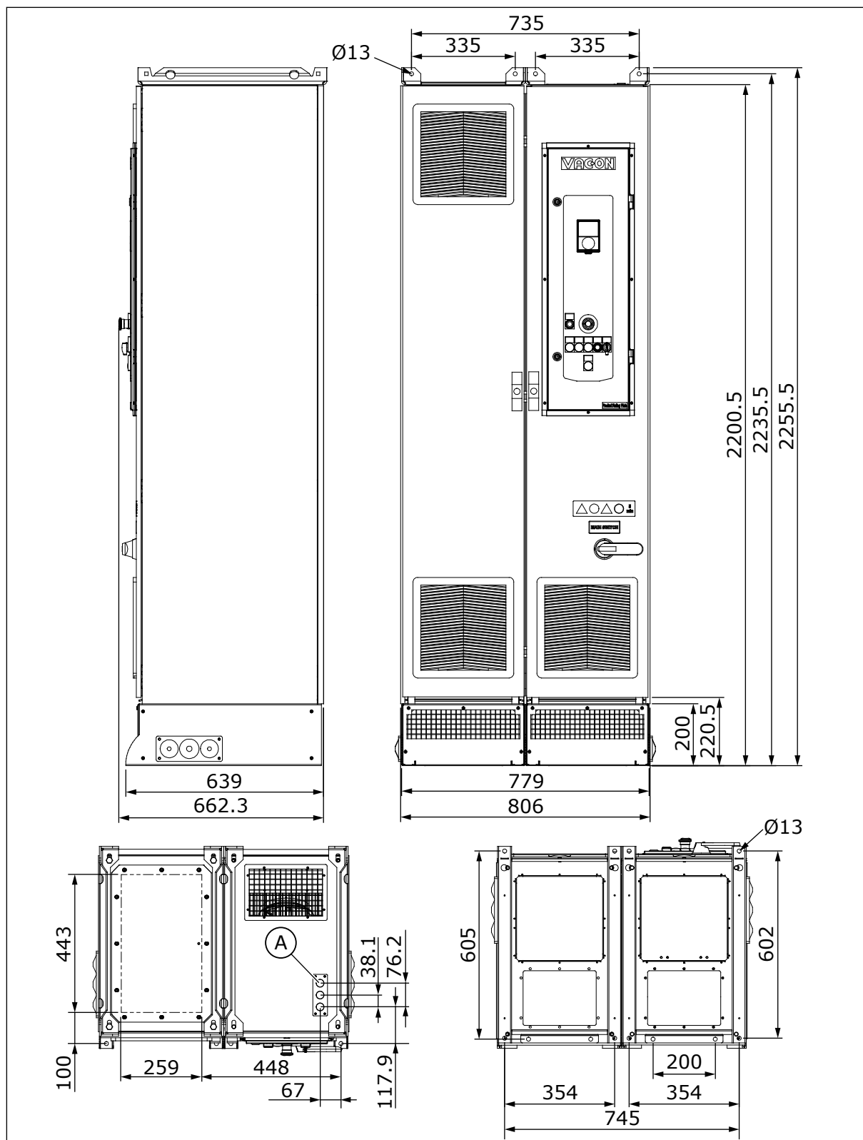
Рис. 12: Габариты шкафа с дополнительными кабелями сверху, MR8, [мм], NAM
