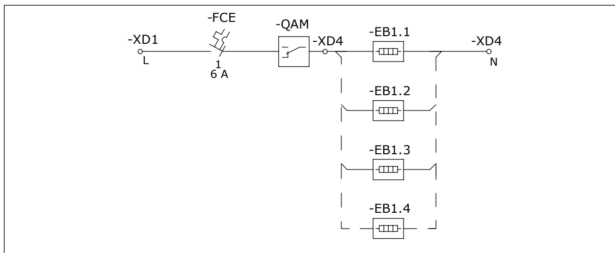
Рис. 16: Нагреватель шкафа
